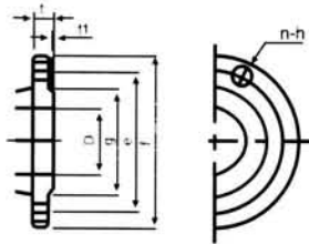
FLANGE JIS 10K RF
